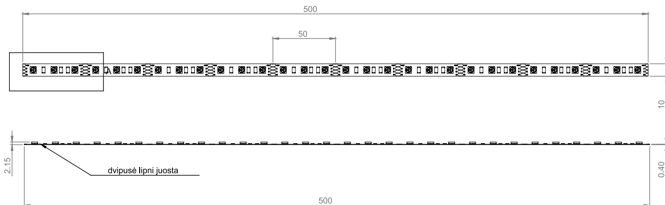
DETALĖ A
