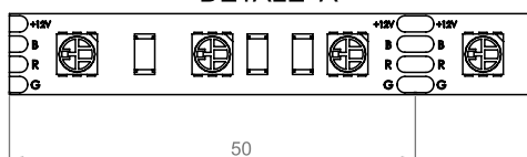
DETALĖ A
