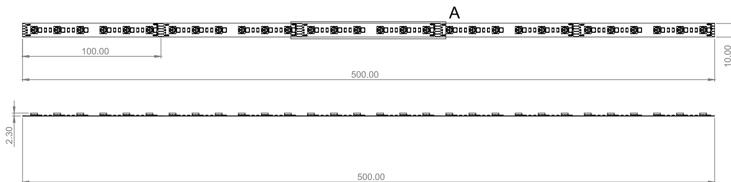
DETALĖ A
